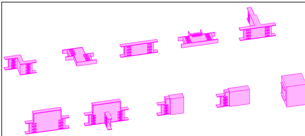
「CADEWA Smart V7」で追加搭載した共同カイツック株式会社製のバスダクト部材
