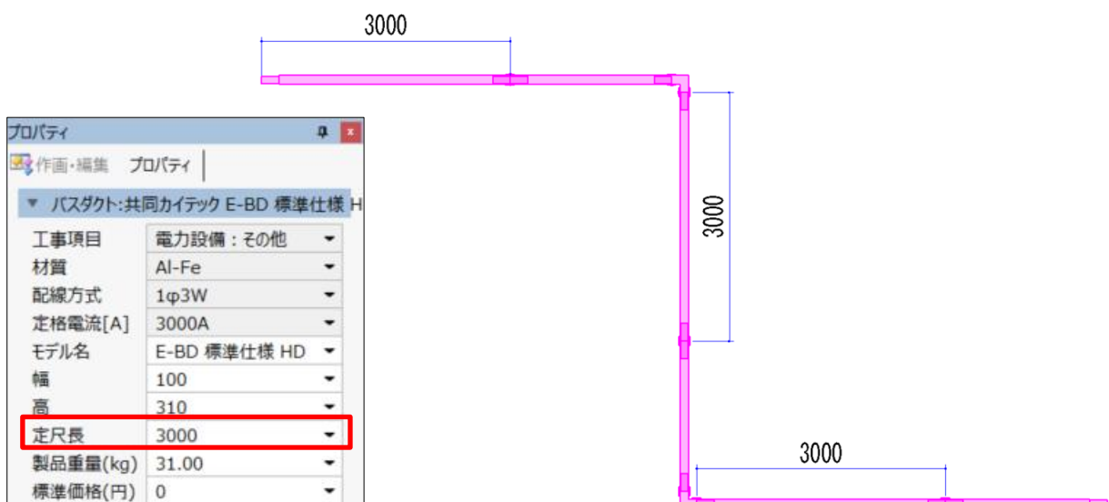
バスダクト定尺ルートの自動作画イメージ
